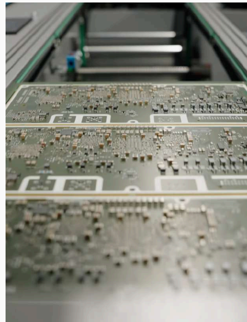
Pájení v reflow peci
