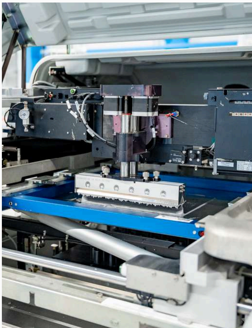
Nanášení pájecí pasty
